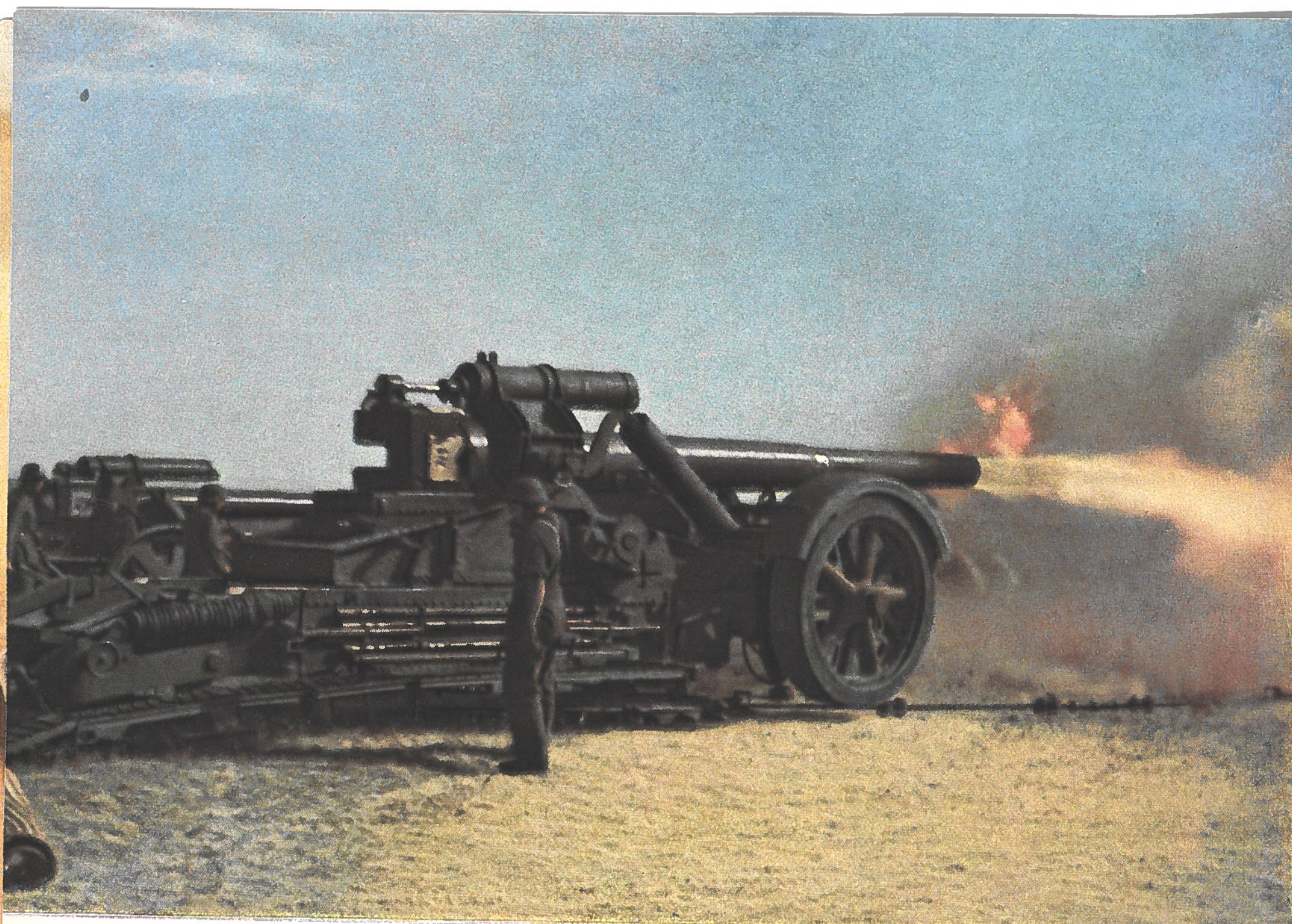
Batterie lourde en tir direct.
